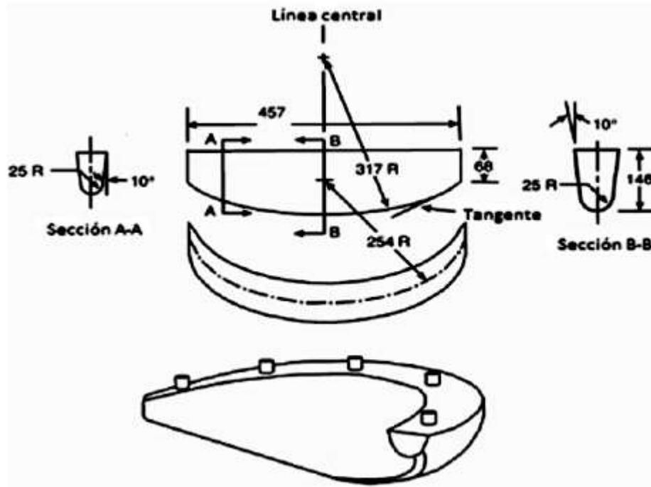
Figura 2 A.- Esquema del bloque metálico patrón usado en la prueba de resistencia de la ceja al desmontaje del rin
